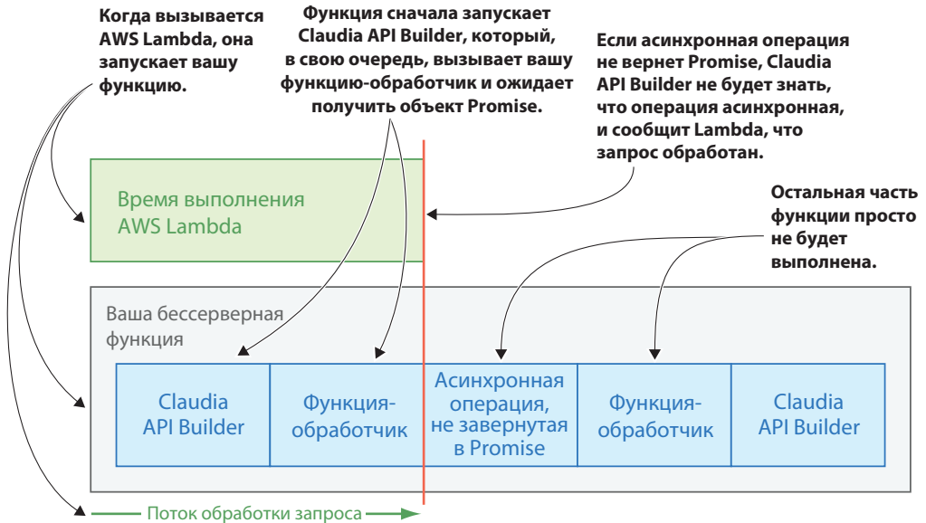
Рис. 4.6. Визуальное представление порядка выполнения функции Lambda, когда асинхронная операция не заключена в Promise
