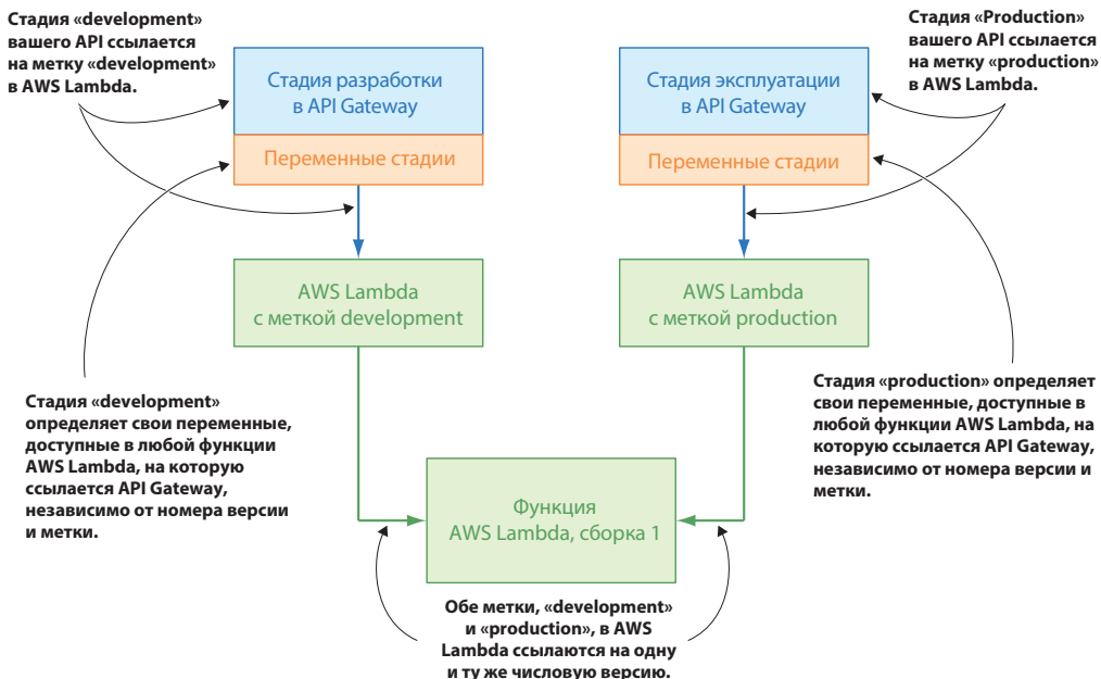
Рис. 14.6. Как работают переменные стадий в API Gateway
