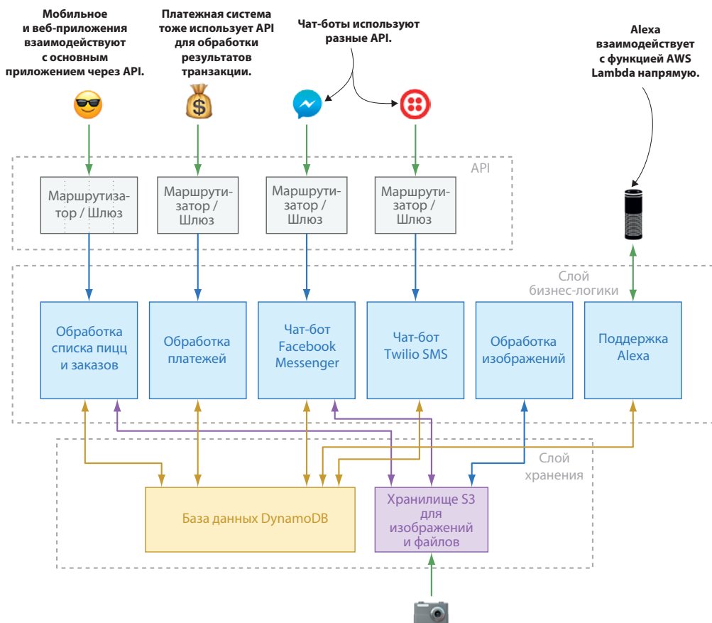
Рис. 14.1. Диаграмма, иллюстрирующая бессерверные службы в приложении для тетушки Марии и отношения между ними
