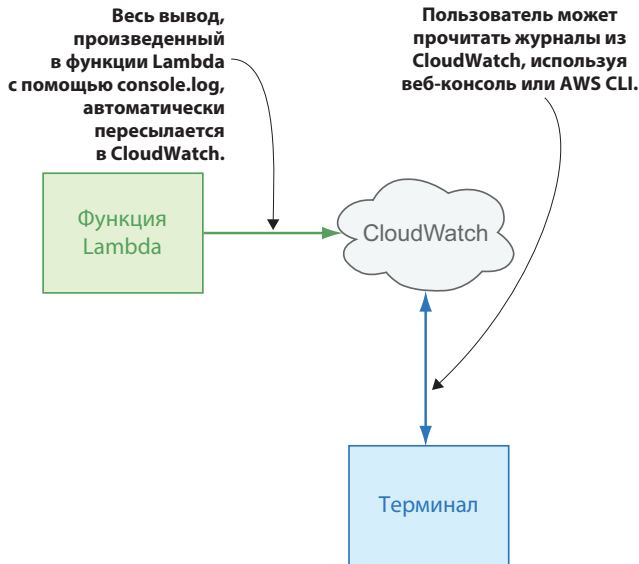
Рис. 5.1. AWS Lambda посылает вывод console.log непосредственно в CloudWatch
