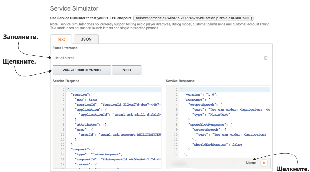
Рис. В.32. Тестирование сценария
