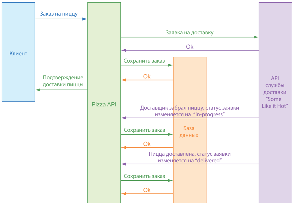
Рис. 4.2. Диаграмма, иллюстрирующая порядок взаимодействий обработчика createOrder с Some Like It Hot API и базой данных
