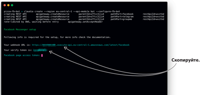
Рис. В.8. Настройка чат-бота Facebook Messenger с использованием Claudia Bot Builder
