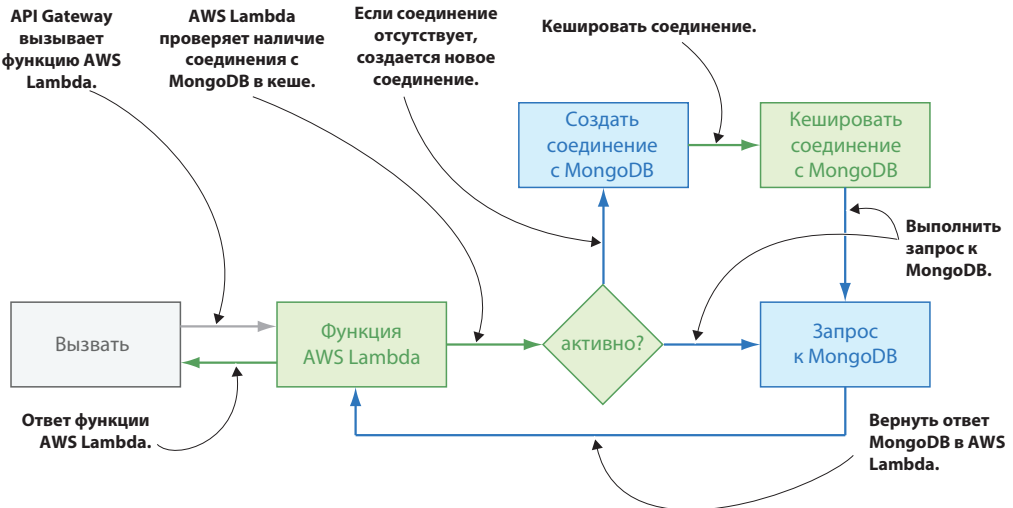
Рис. 13.3. Процесс подключения к базе данных MongoDB и кеширования активного соединения
