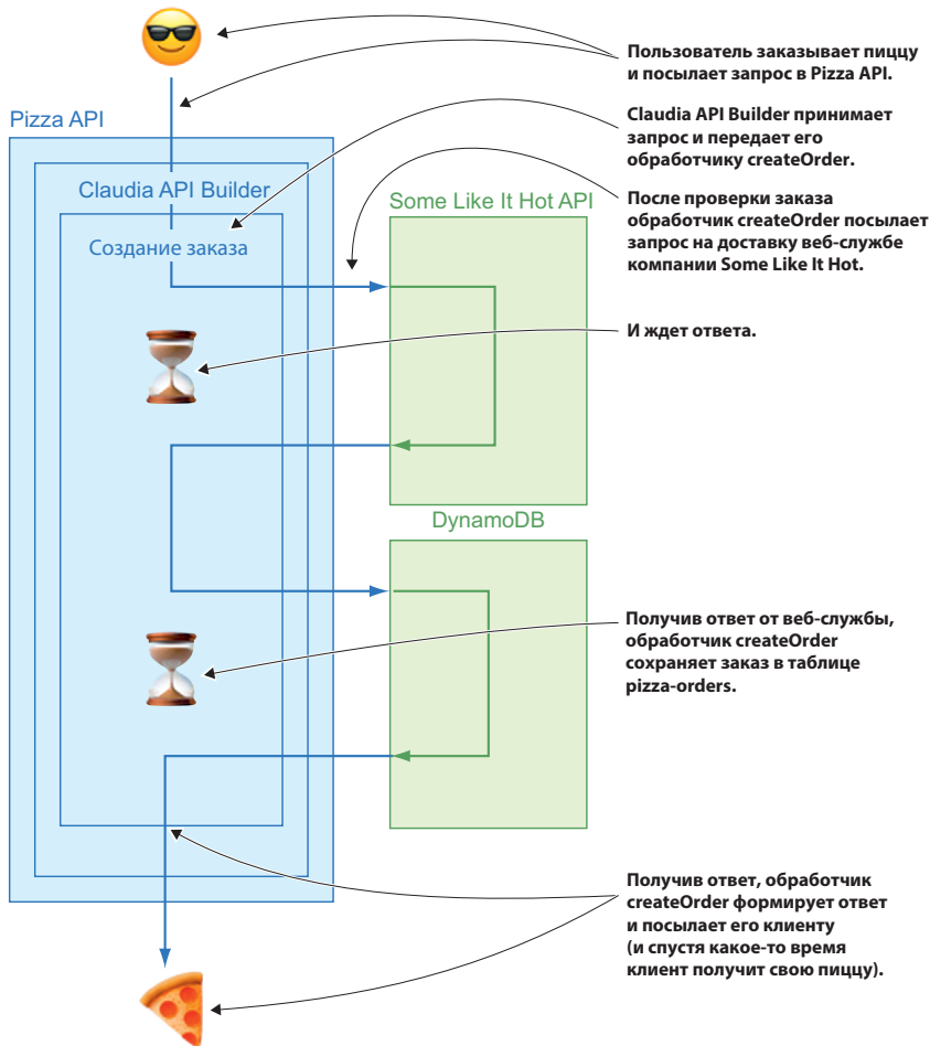
Рис. 4.3. Процесс от заказа до доставки
