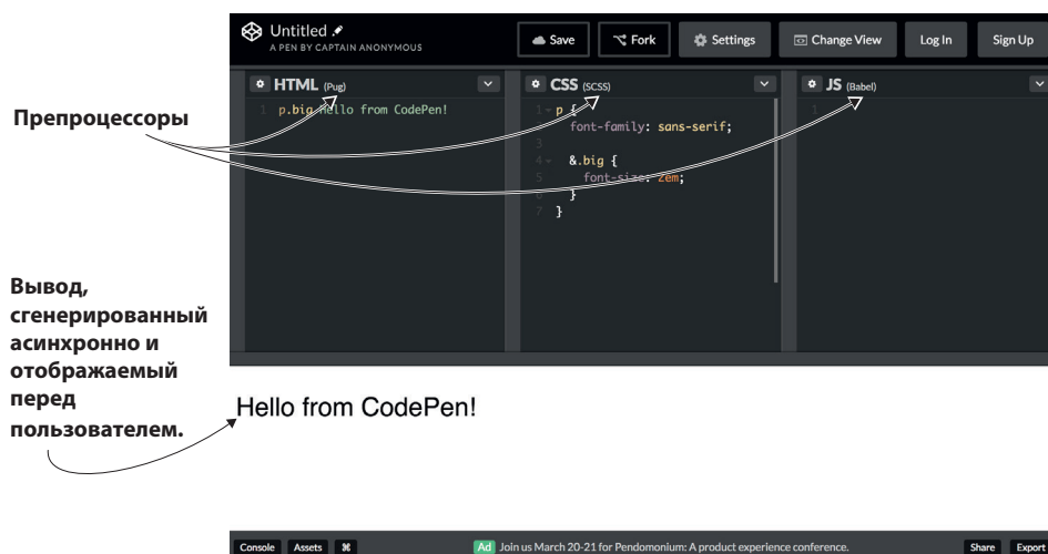
Рис. 15.2. Препроцессоры CodePen
