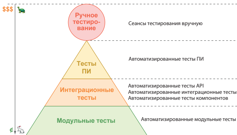
Рис. 11.1. Пирамида тестирования
